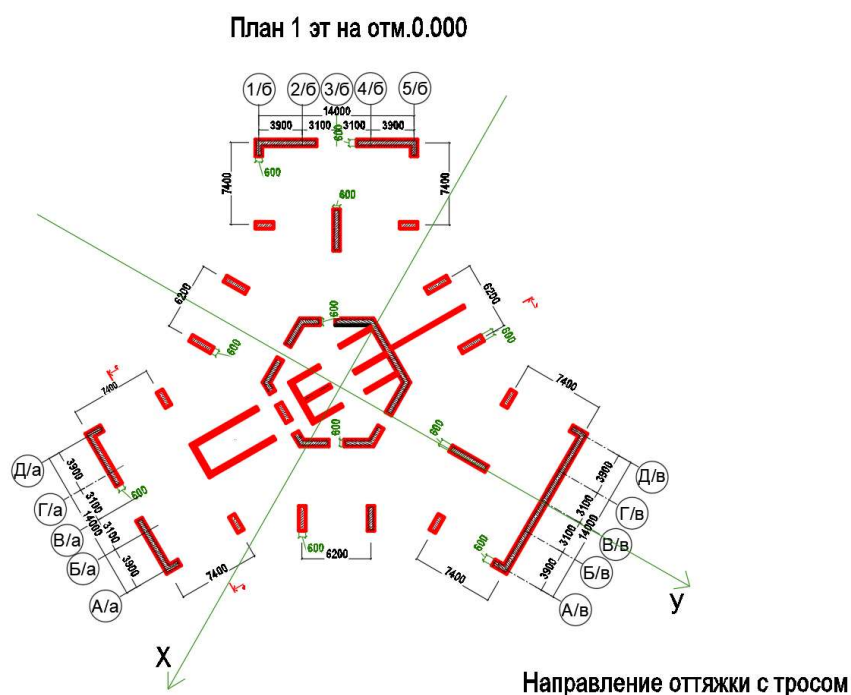
Рисунок 24 – Планы этажей экспериментального здания
