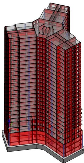
Рисунок С.2 – Общий вид расчетной схемы
