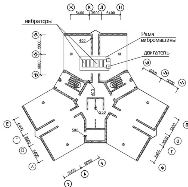
Рисунок 15 – Схема расположения вибрмашины на перекрытии
