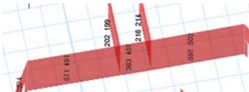
Рисунок С.15 – Фрагмент армирования стены (ДЖМ) на отм. 0.000 м до отм. 4.95 м по оси Г/б (площадь полной арматуры)
