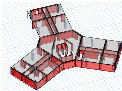
Рисунок С.3 – Схема каркаса подвальных этажей
