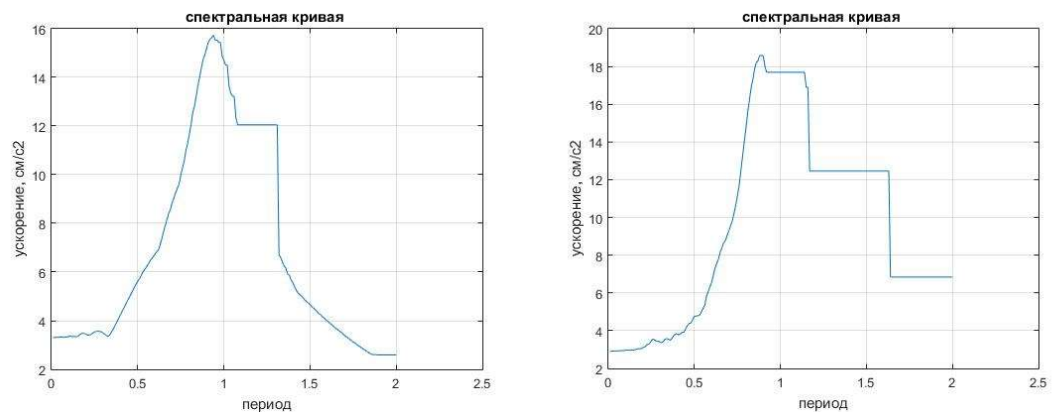
Рисунок 32 – Спектральная кривая акселерограммы канала р3 и р4
