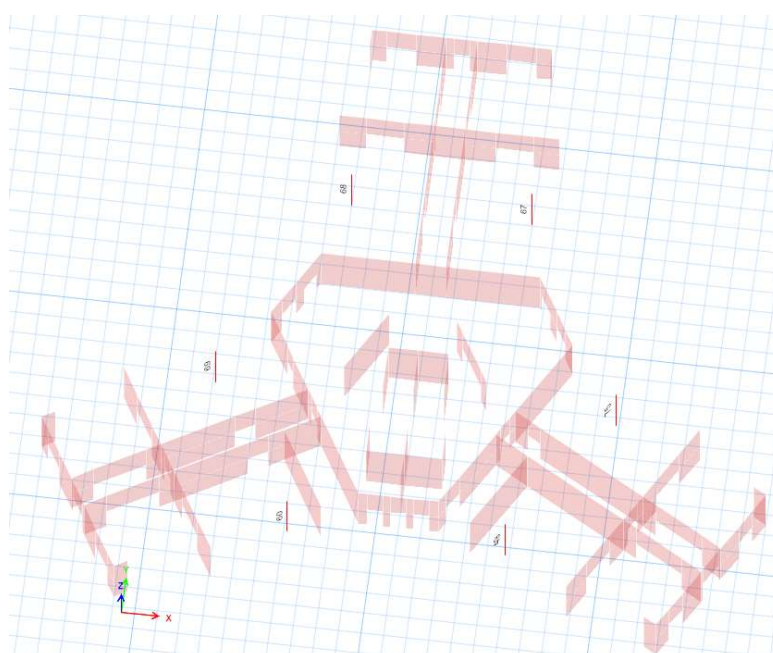
Рисунок С.7 – Армирование колонны на отм. 0.000м до отм. 4.95 м (Площадь полной арматуры)
