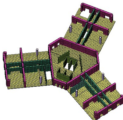
Рисунок 35 – Общий вид здания
