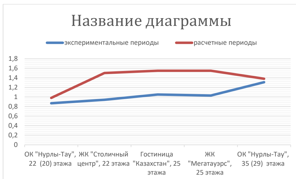
Рисунок 34 – Диаграмма «высота (число этажей) и периоды собственных колебаний» для высотных зданий
