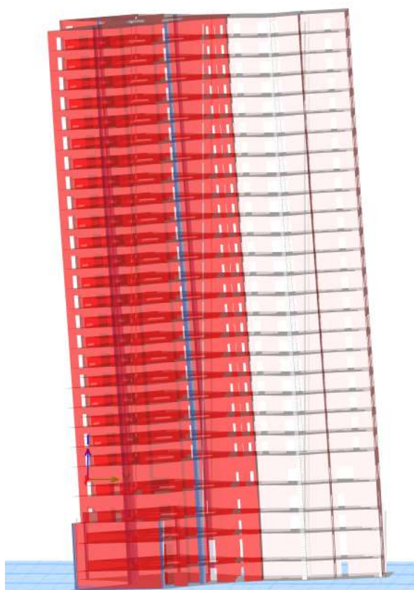
Рисунок С.4 – Схема каркаса надземных этажей
