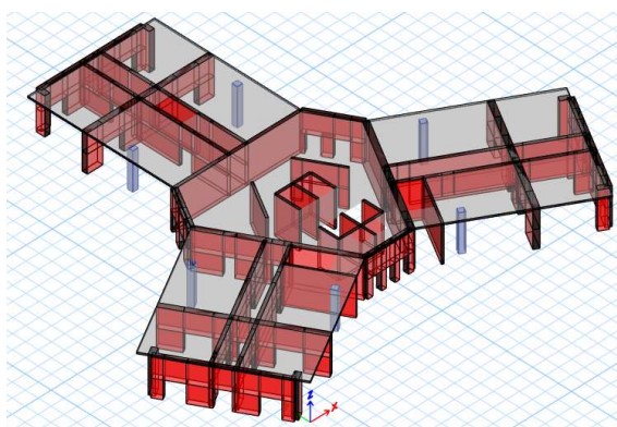
Рисунок С.4 – Схема каркаса надземных этажей
