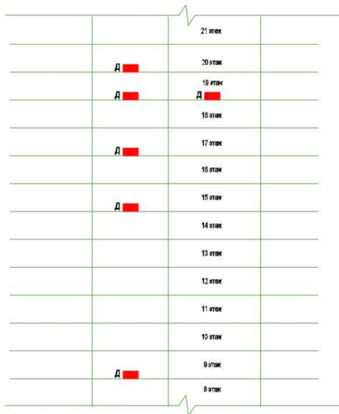
Рисунок 28 – Схема расположения датчиков по высоте здания
