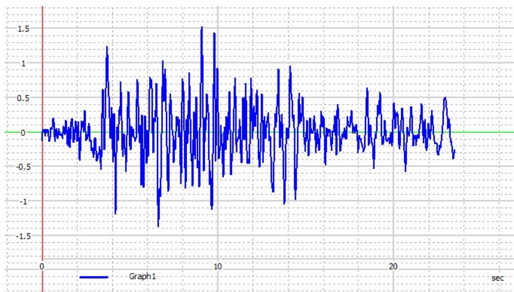
Рисунок 37 – График радиального компонента (акселерограмма Aks. 24 - Kern Country – 21.07.52г, R=41, M=7.2 по X).
