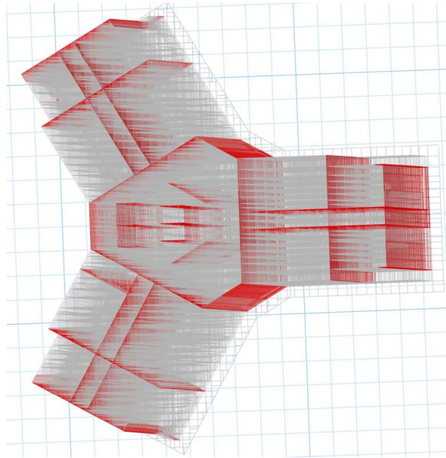
Рисунок С.5 – Первая форма колебаний T=1,02с (поступательная)
