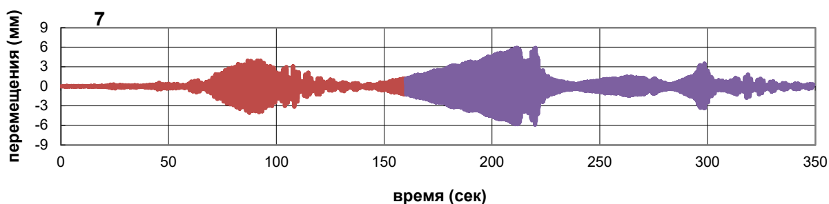
Рисунок 21 – Записи колебания здания на этапе III-3 в уровне перекрытия над 29 этажом
