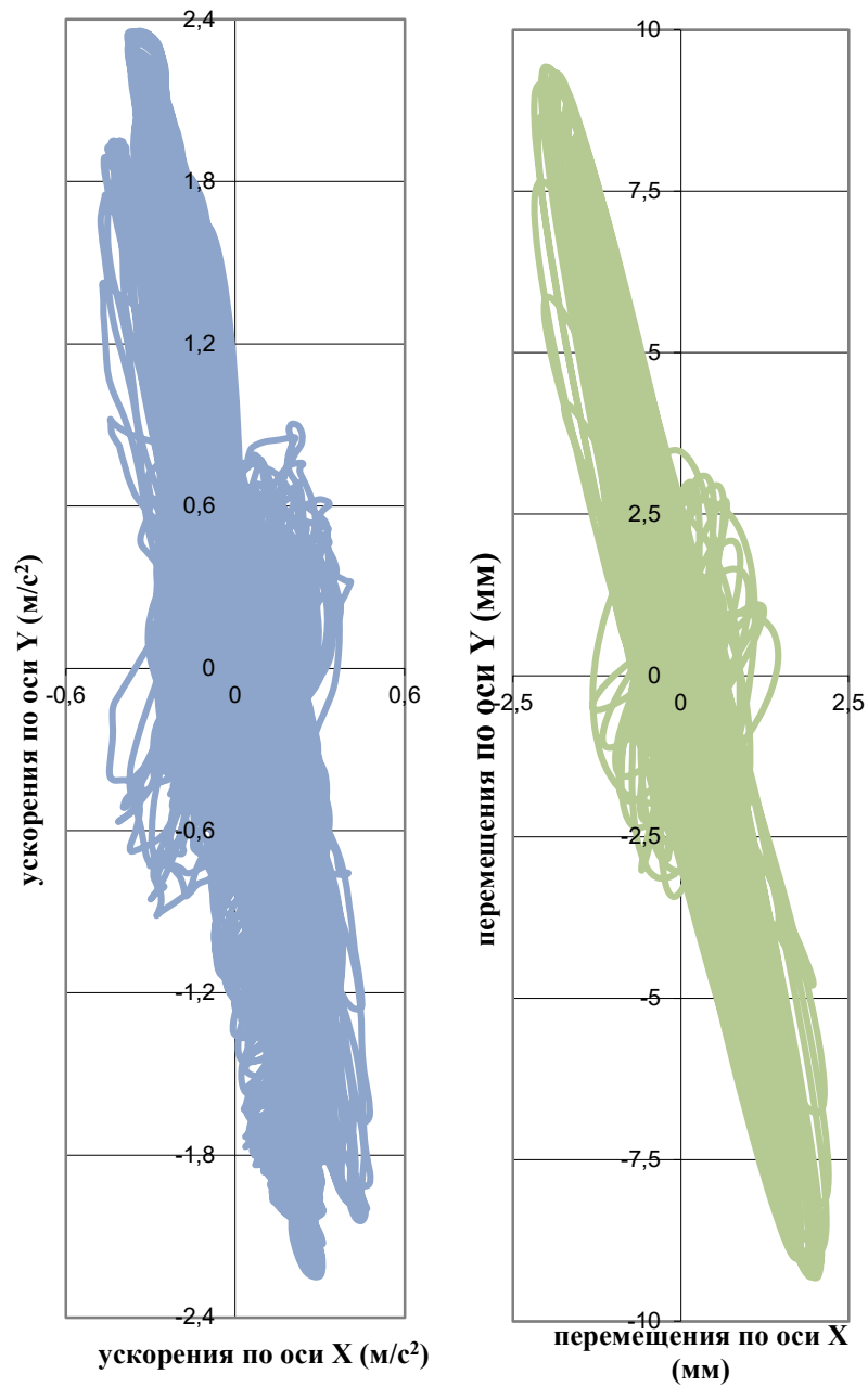
Рисунок 22 – Траекторий движения междуэтажного перекрытия здания над 29 этажом на этапе испытаний III-3
