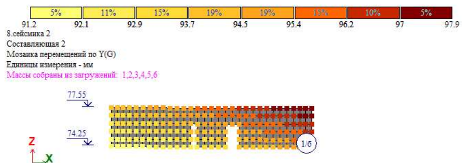
Рисунок 42 – Мозаика перемещений по оси X по инструментальным акселерограммами Aks.7
