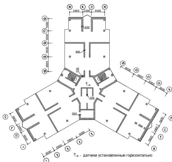
Рисунок 13 – Типовой план высотного монолитного здания
