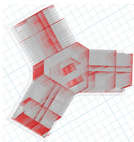
Рисунок С.6 – Вторая форма колебаний T=1,38c (поступательная)
