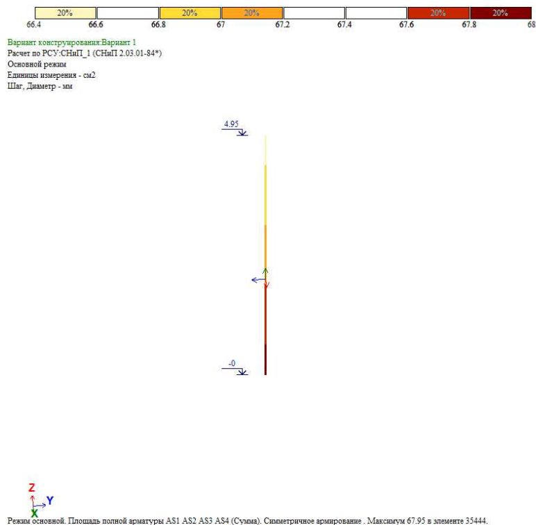
Рисунок Б.7 – Фрагмент колонны по оси 2/а на отм. 0.000м до отм. 4.95 м (площадь полной арматуры, стержень 34814)
