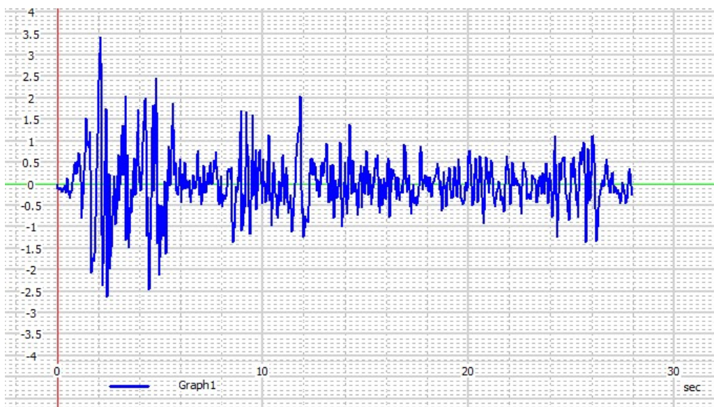
Рисунок 36 – График радиального компонента (акселерограмма Aks. 7 - г. El-Centro- 18.05.40г, R=31, M=6.5 по X)
