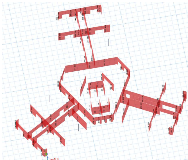
Рисунок С.14 – Фрагмент армирования стены (ДЖМ) на отм. 0.000 м до отм. 4.95 м (площадь полной арматуры)
