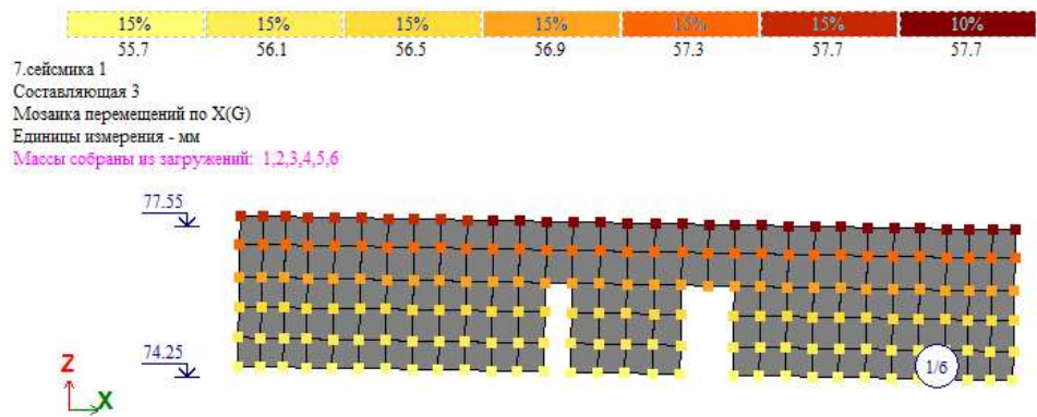
Рисунок 40 – Мозаика перемещений по оси X по спектральному методу
