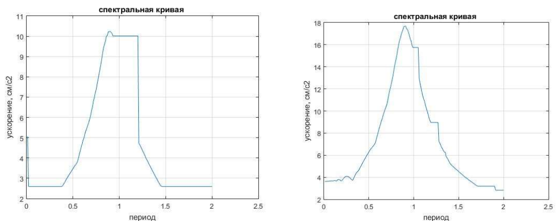
Рисунок 32 – Спектральная кривая акселерограммы канала р3 и р4
