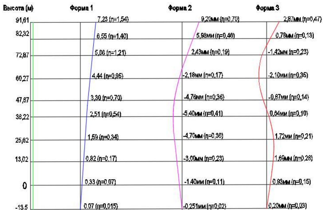
Рисунок 23 – Формы колебаний вертикальной оси здания
