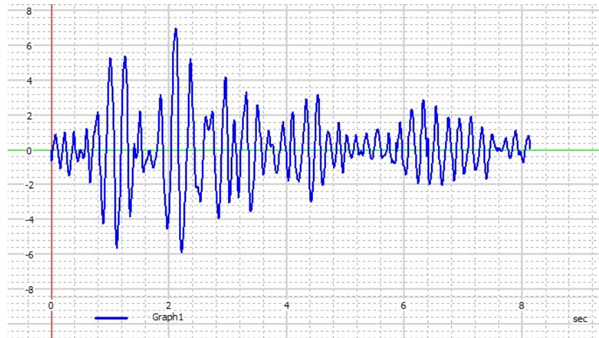
Рисунок 38 – График радиального компонента (акселерограмма Aks.190 Байсорунское -12.11.90г, D=35, H=20, M=6.3 по X)
