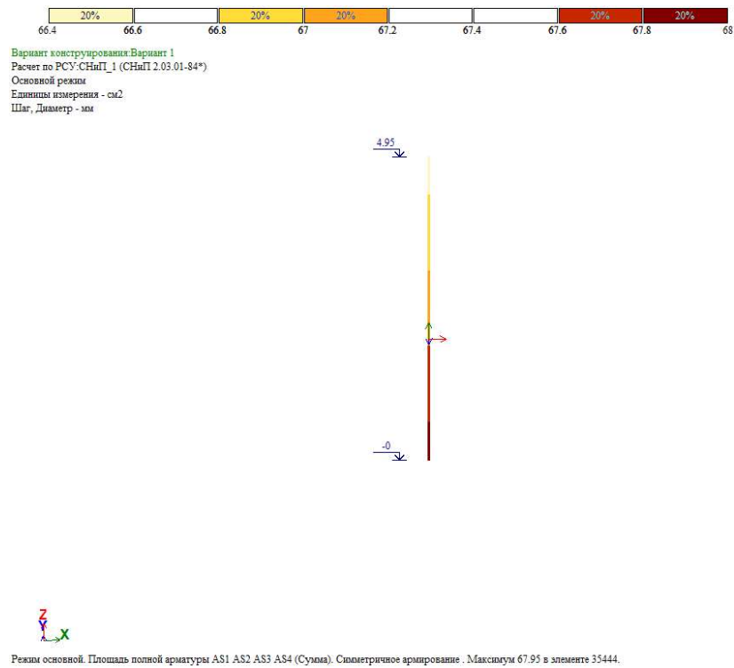
Рисунок Б.6 – Фрагмент колонны по оси Г/в на отм. 0.000м до отм. 4.95 м (площадь полной арматуры, стержень 35444)
