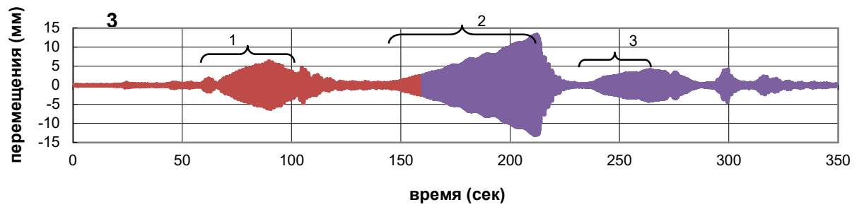
Рисунок 20 – Записи колебания здания на этапе III-3 в уровне перекрытия над 29 этажом
